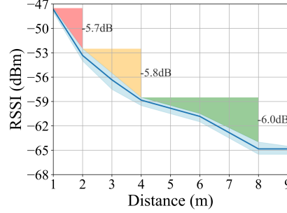
Figure 5: Tag-to-reader RSSI.
