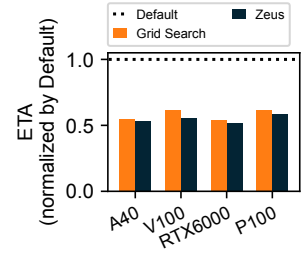
Figure 14: Normalized ETA w.r.t. GPU models.
