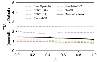
(b) TTA
