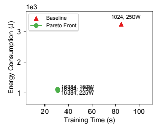
(f) NeuMF
