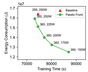
(d) ResNet-50
